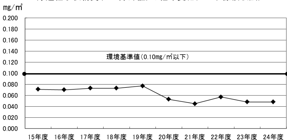
浮遊粒子状物質(2%除外値)の経年変化(ベータ線吸収法)
