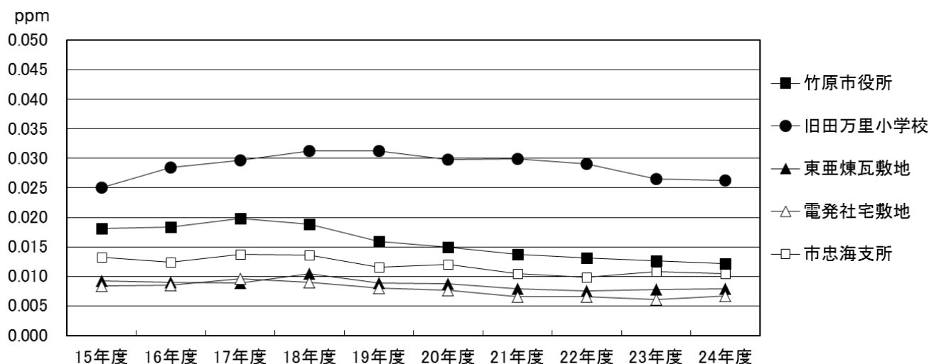
窒素酸化物(年平均値)の経年変化(NG-KN-S法)
