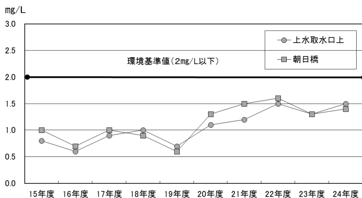
賀茂川水系BOD (75%値) の経年変化
