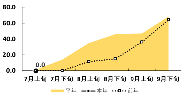
紋枯病 発生地点率(県全域27地点)
