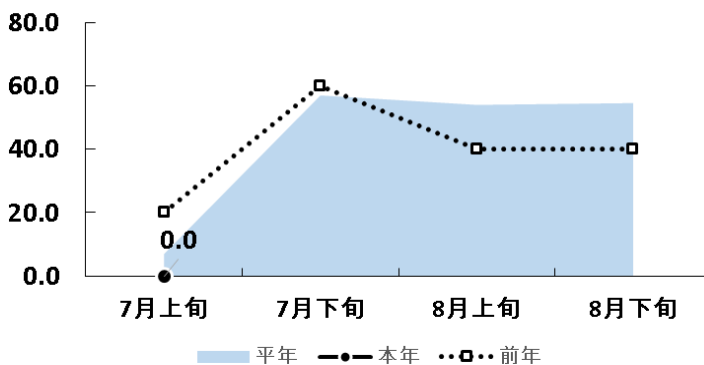
葉いもち 発生地点率(南部 5地点)
