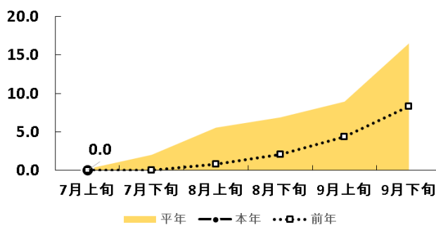
紋枯病 発生株率(県全域27地点)
