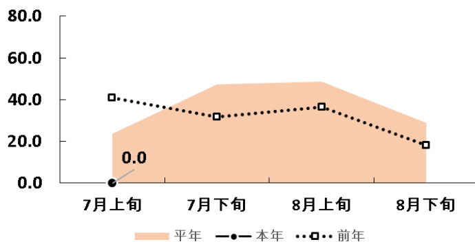
葉いもち 発生地点率(南部 5地点)
