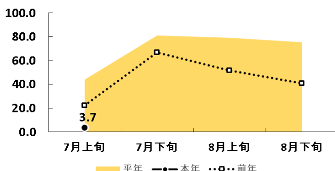
セジロウンカ 発生地点率(県全域27地点)
