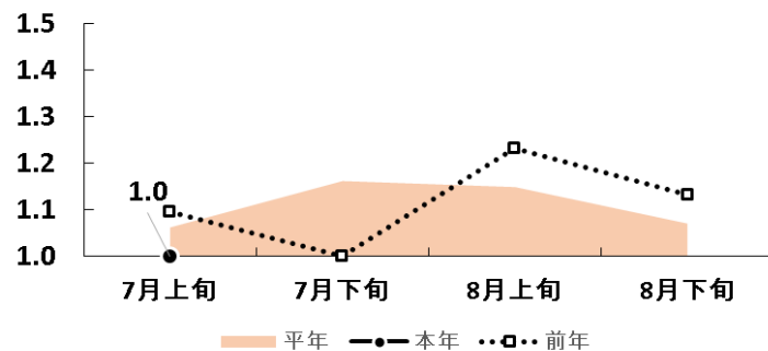
葉いもち 発生程度(南部 5地点)
