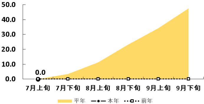
トビイロウンカ 発生地点率(県全域27地点)
