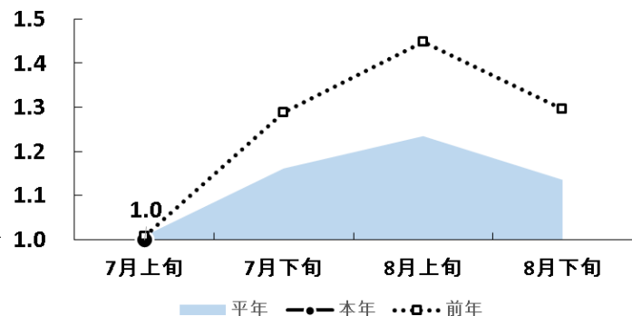
葉いもち 発生程度(南部 5地点)
