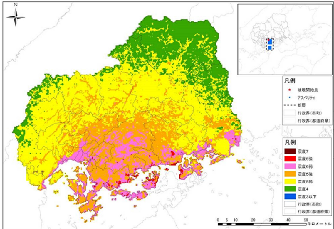
安芸灘～伊予灘～豊後水道の地震 (北から破壊)
