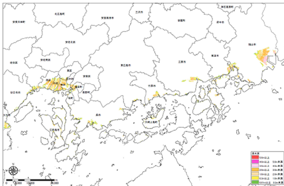
南海トラフ巨大地震（ケース 1）
