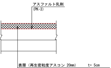
打ち換え部 S=1:10
