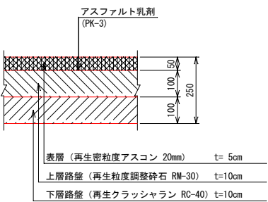
すり付け部 S=1:10
