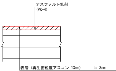
オーバーレイ部 S=1:10
