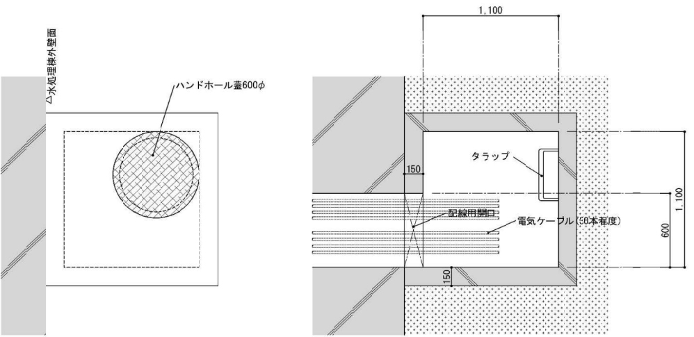
耐水化前 平面図(地上) 1/40
