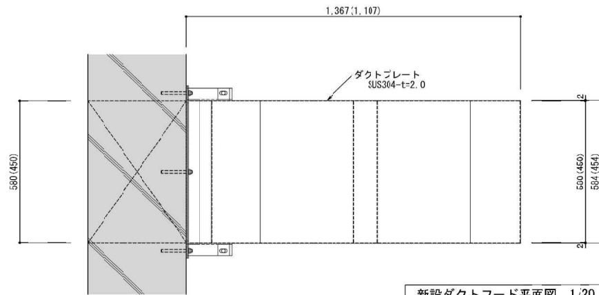
新設ダクトフード平面図 1/20
