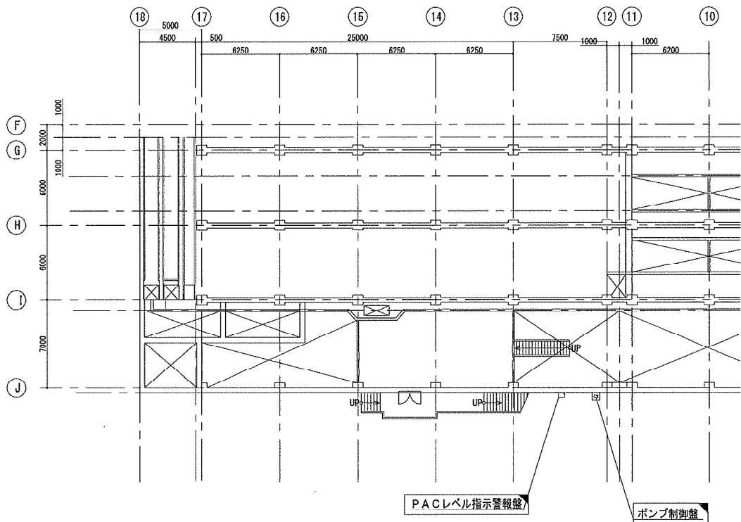
平面図 1/400
