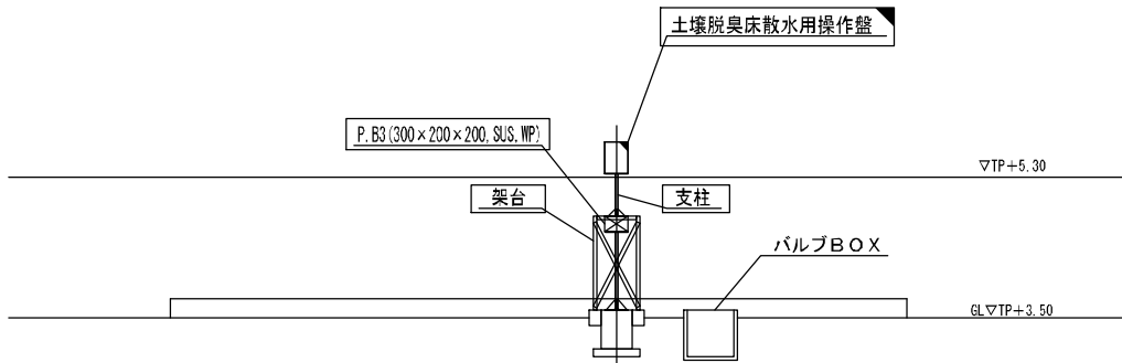
土壌脱臭床 断面図 1/100
