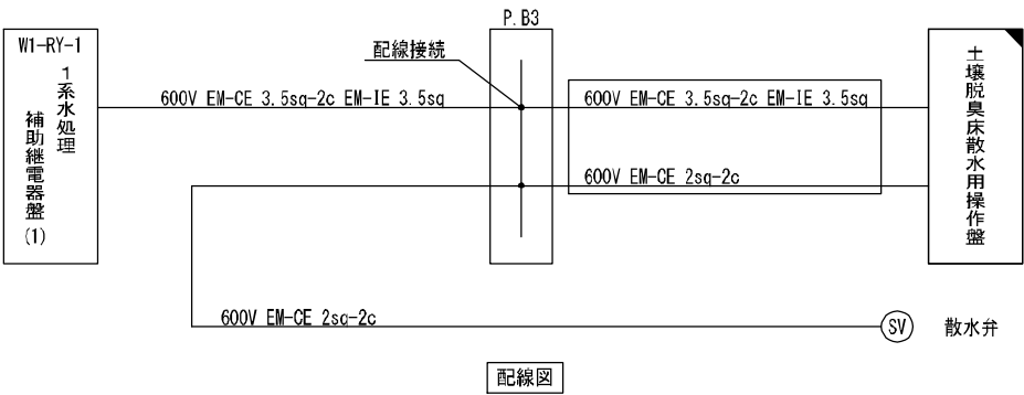
配線図
