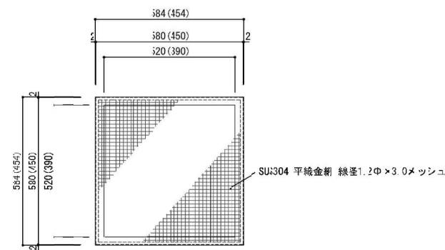
B-B 矢視図 1/20
