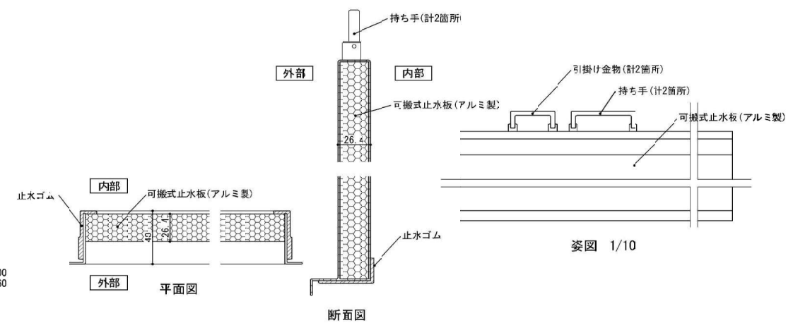
断面図
