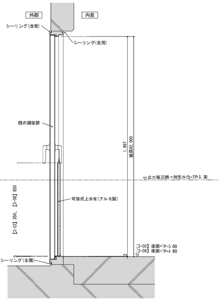
耐水化後 断面詳細図 1/20
