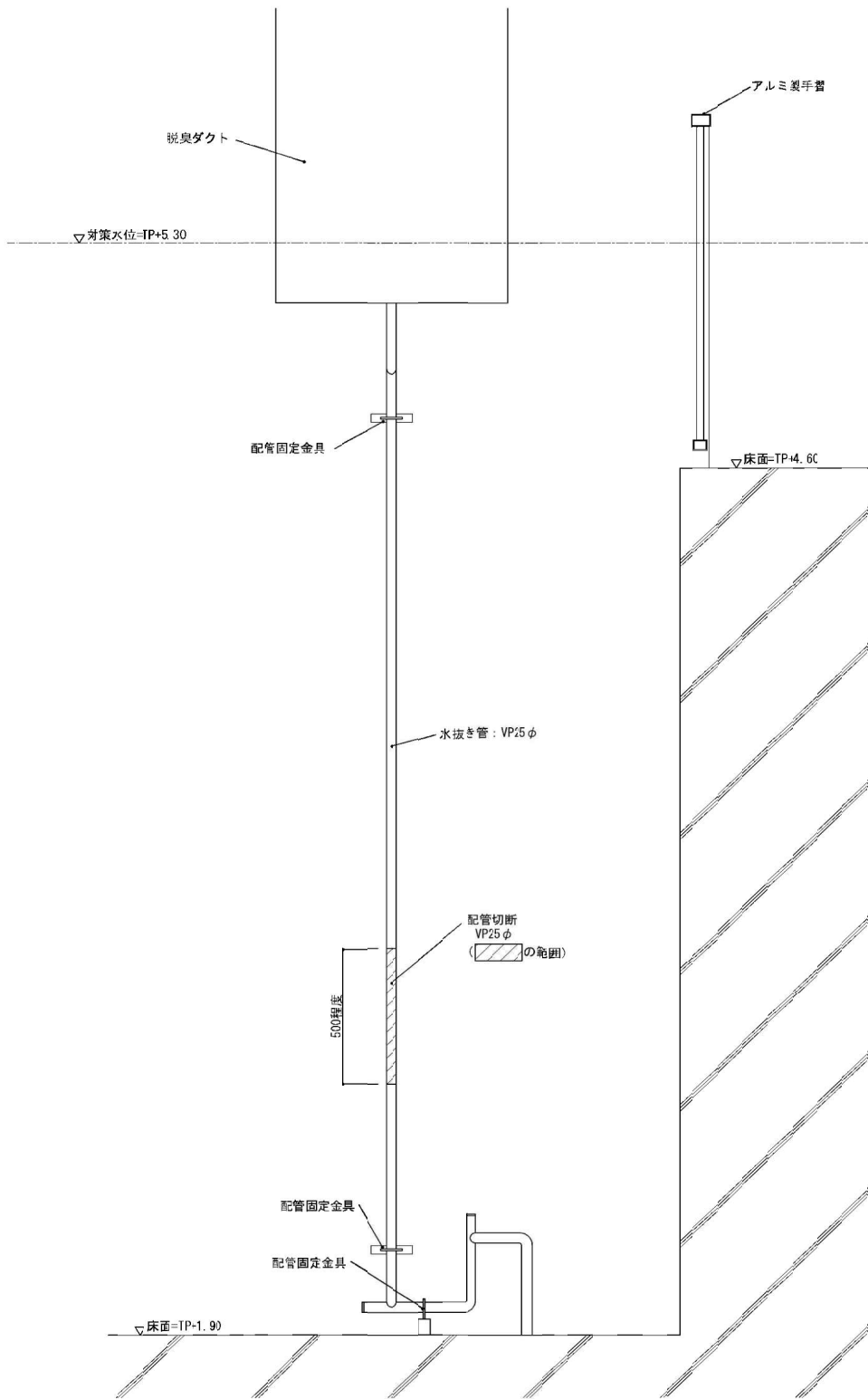
耐水化前 正面図 1/20
