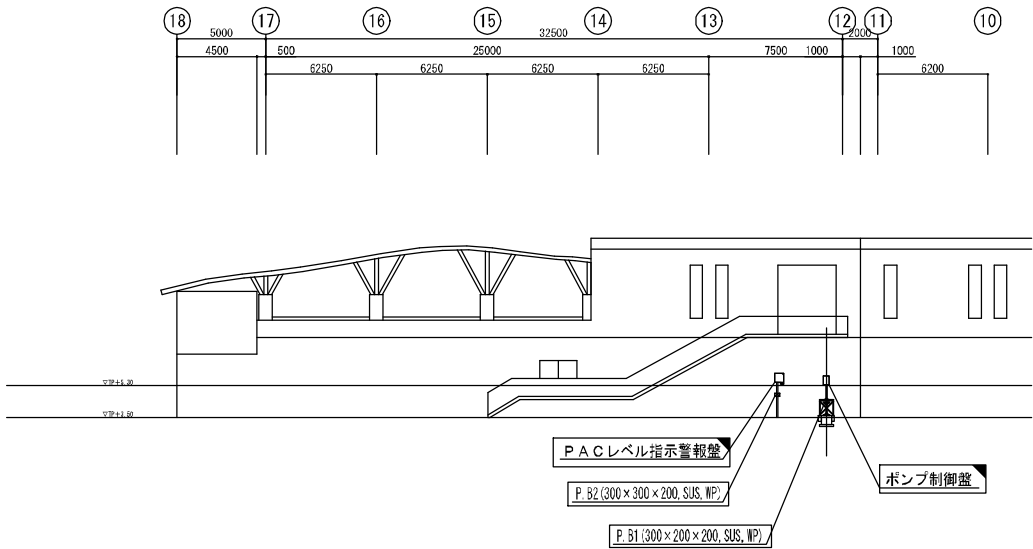
立面図 1/400
