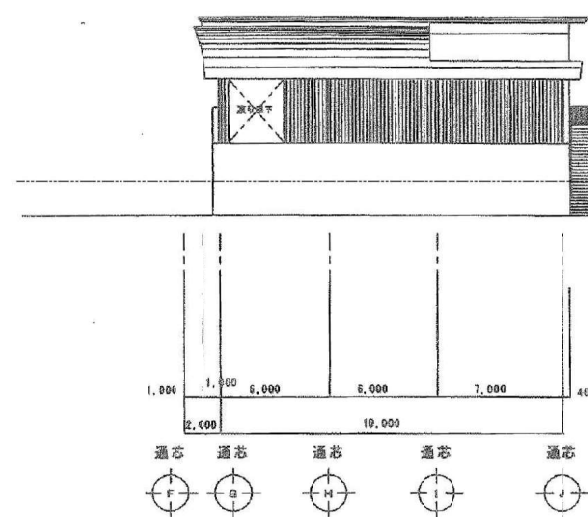
水処理棟 南立面図 1/400
