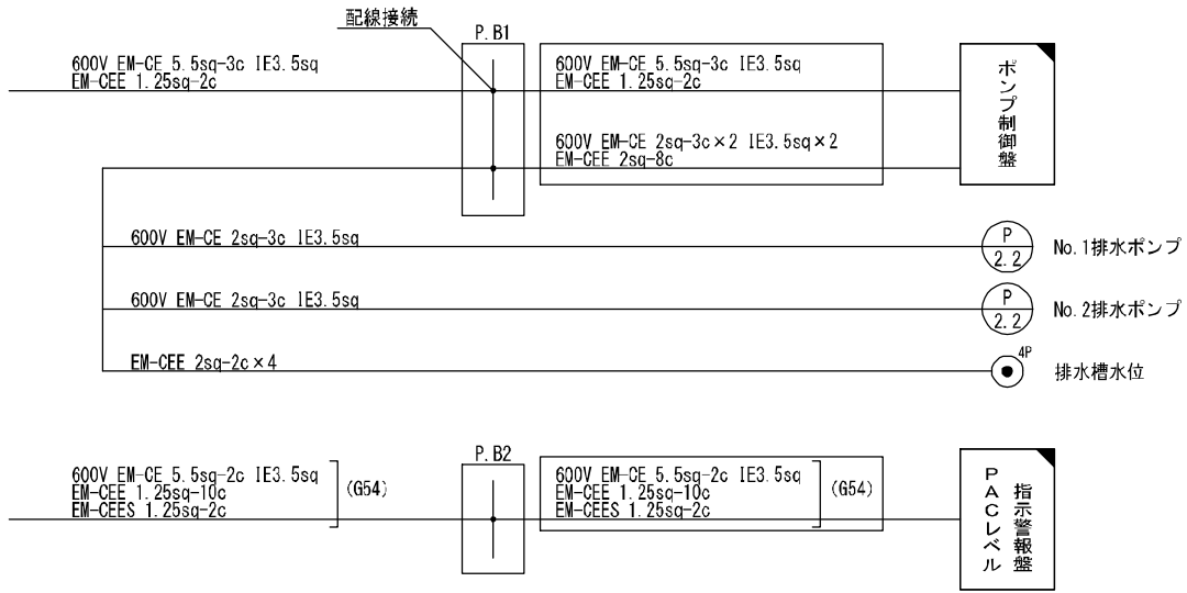
配線図
