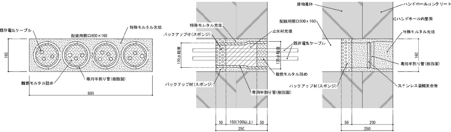
耐水化後 貫通部密閉詳細図 1/10
