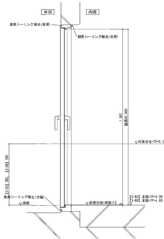
耐水化前 断面詳細図 1/20
