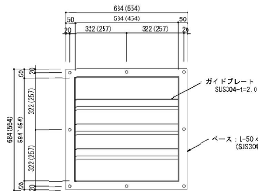
A-A 矢視図 1/20
