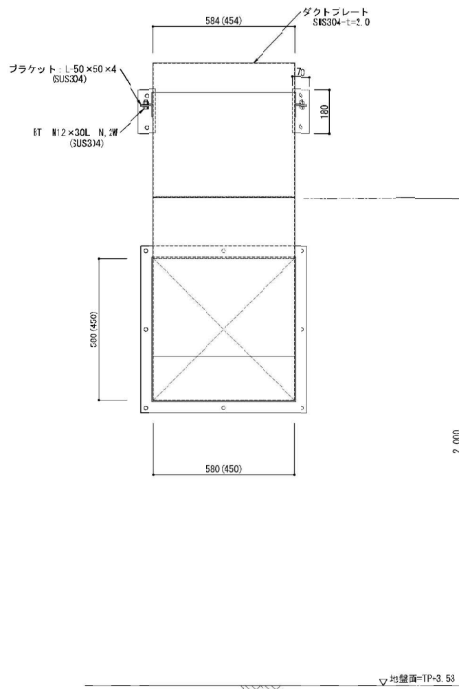
新設ダクトフード正面図 1/20
