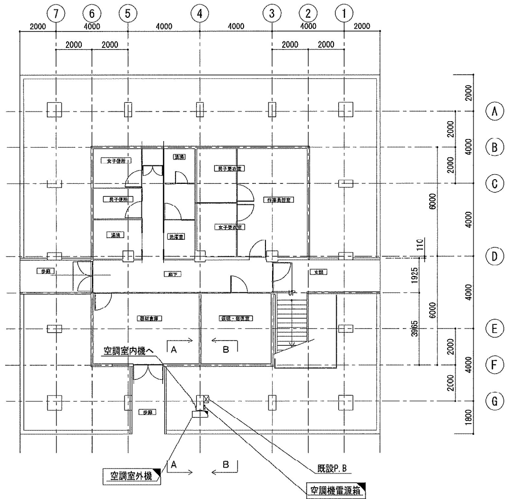
1階 平面図 1/200
