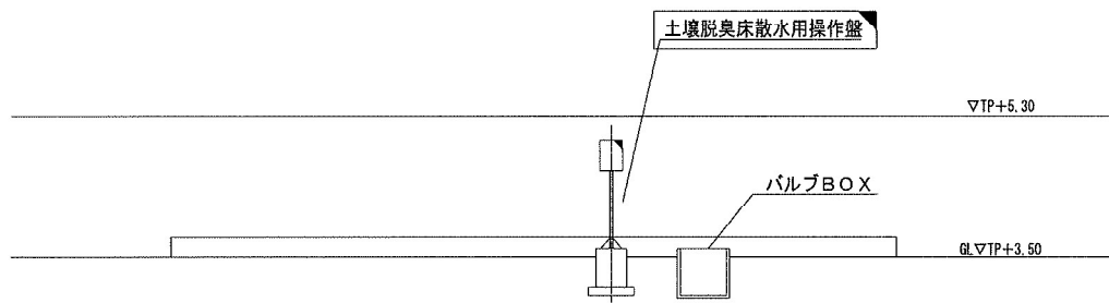
土壌脱臭床 断面図 1/100
