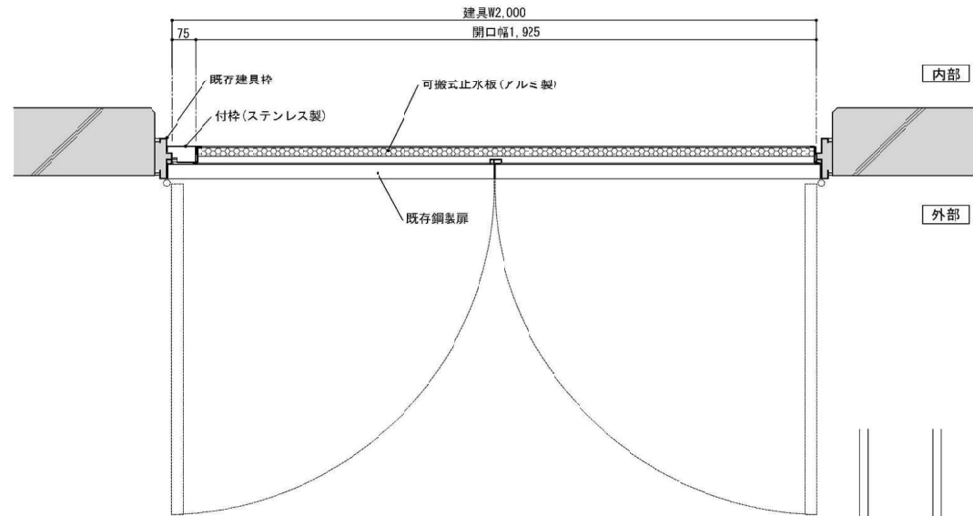
耐水化後 平面詳細図 1/20
