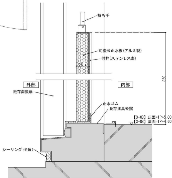
耐水化後 断面詳細図 1/4
