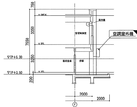
A-A 断面 1/200
