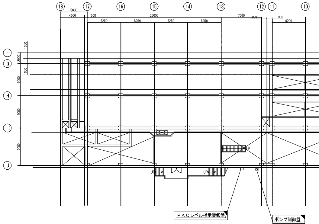
平面図 1/400
