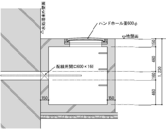
耐水化前 断面図 1/40
