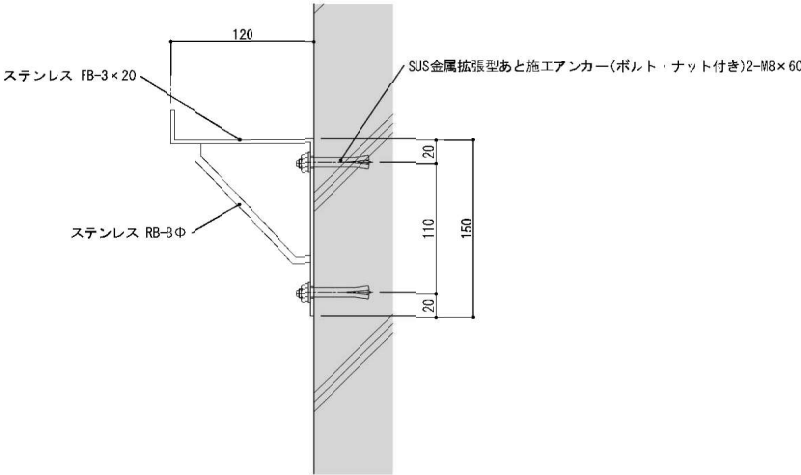
フック：側面図 1/6
