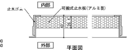
平面図
