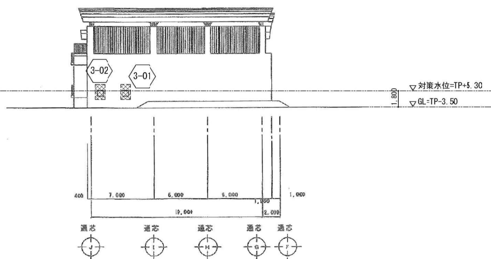
水処理棟 北立面図 1/400
