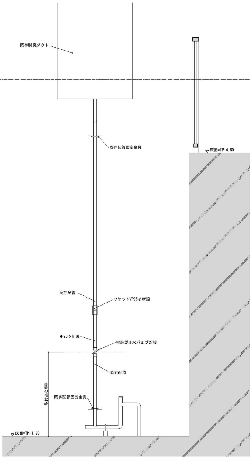
耐水化後 正面図 1/20
