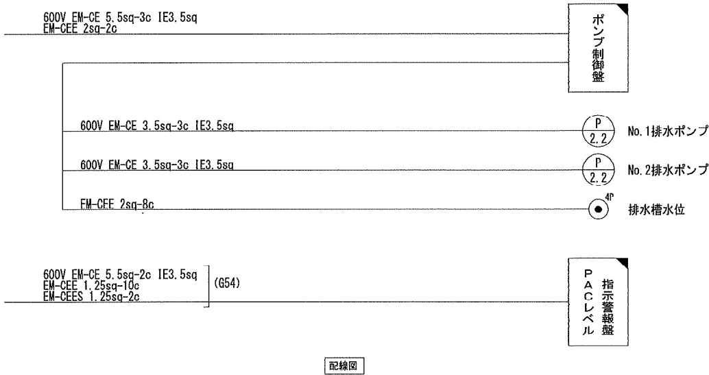
配線図
