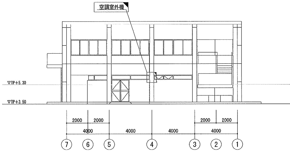
北面 立面図 1/200
