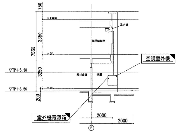
A-A 断面 1/200
