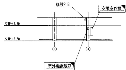
B-B 断面 1/200
