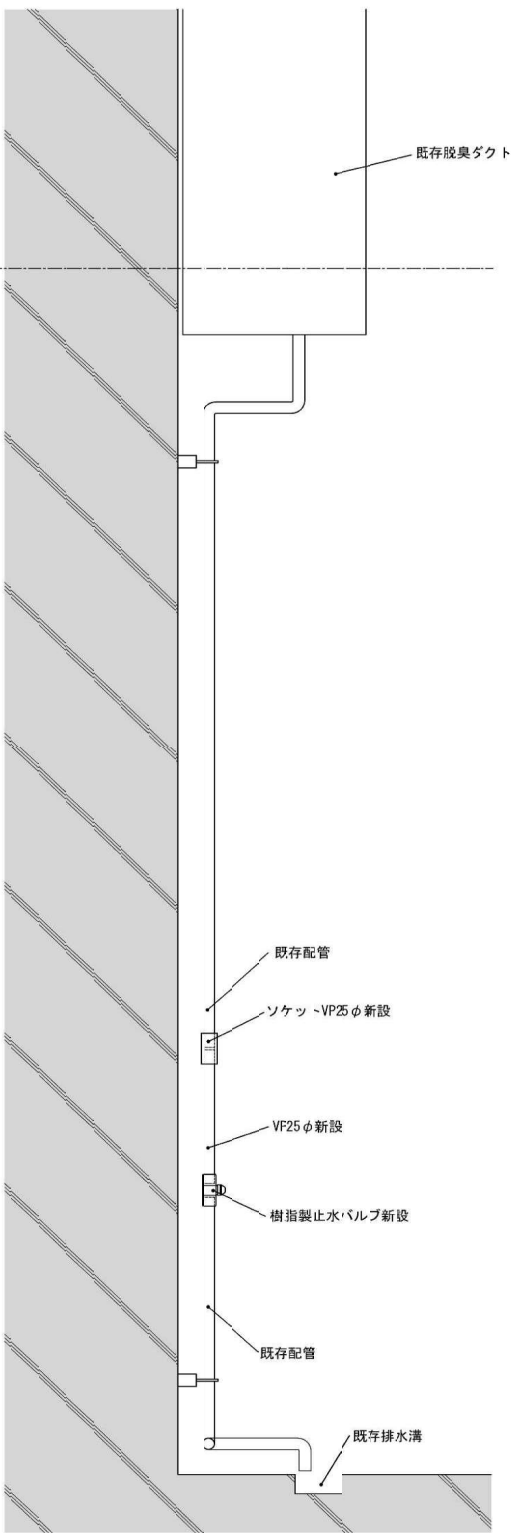
耐水化後 側面図 1/20
