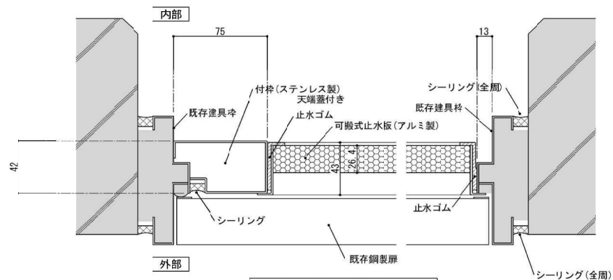
耐水化後 平面詳細図 1/4
