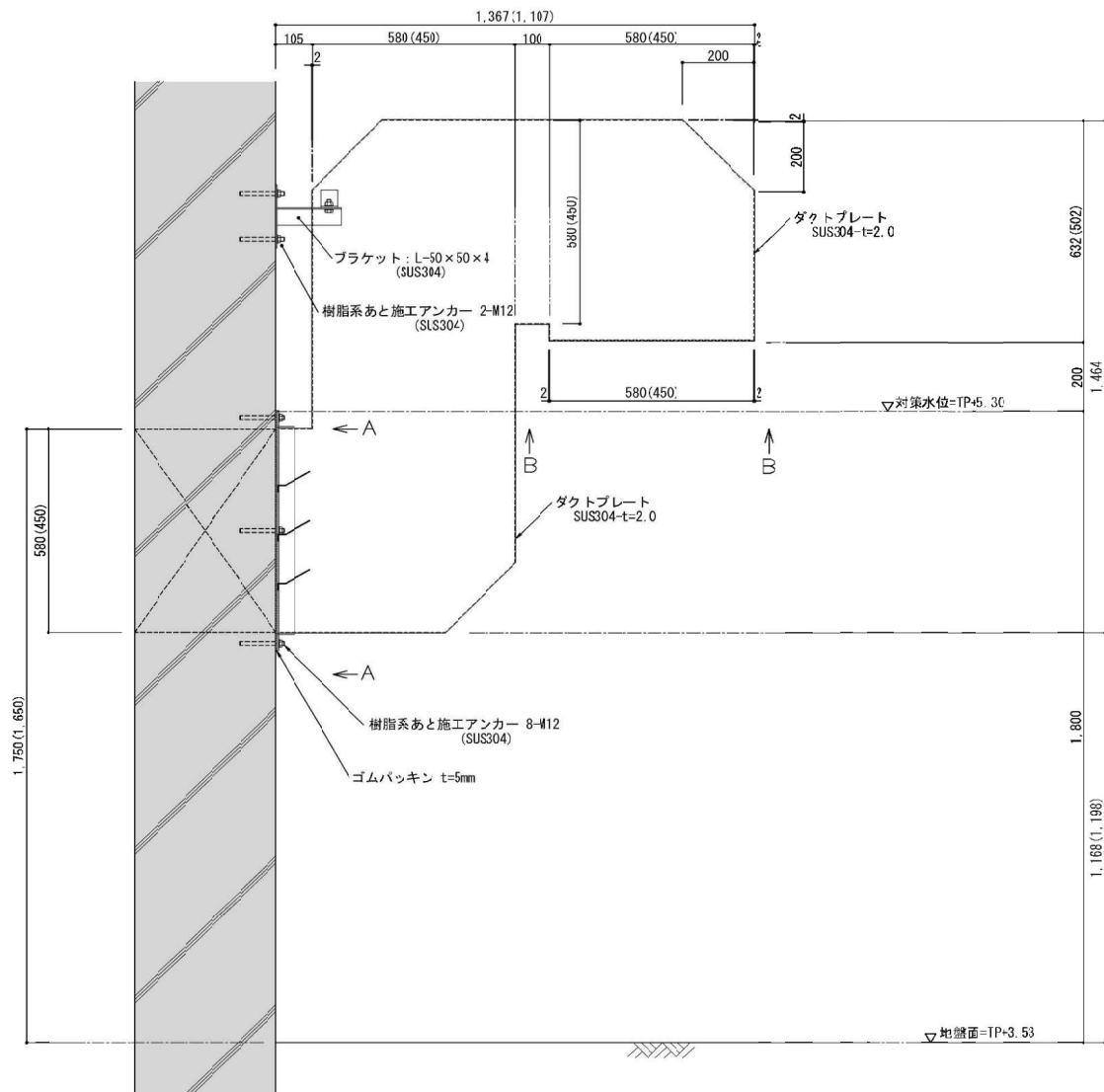
新設ダクトフード断面図 1/20
