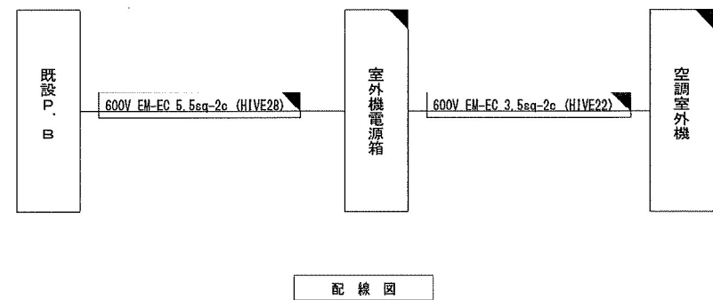
配線図
