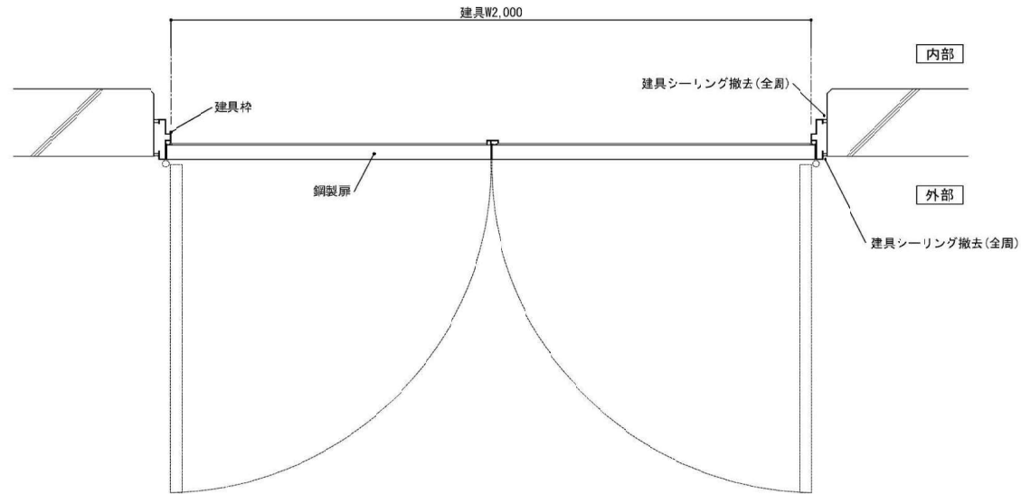
耐水化前 平面詳細図 1/20
