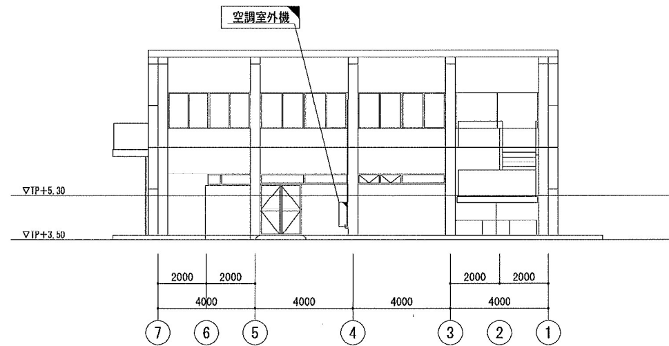
北面 立面図 1/200
