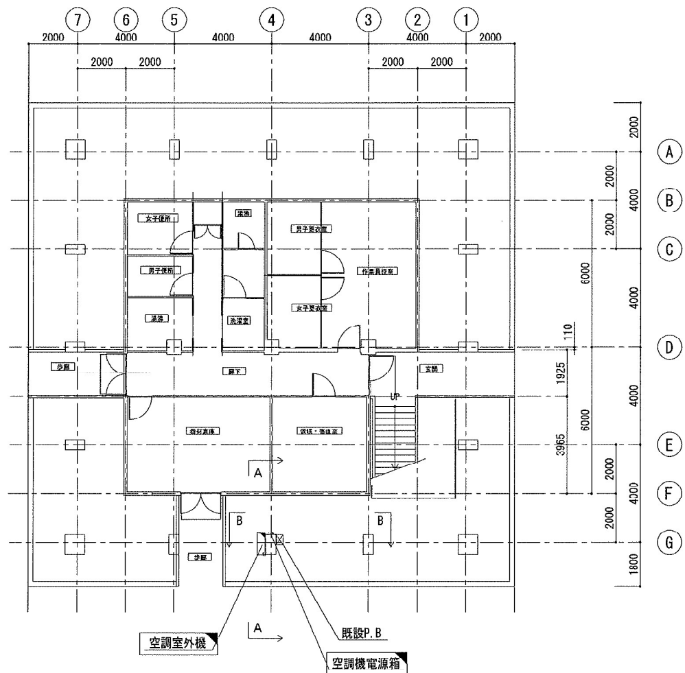
1階 平面図 1/200
