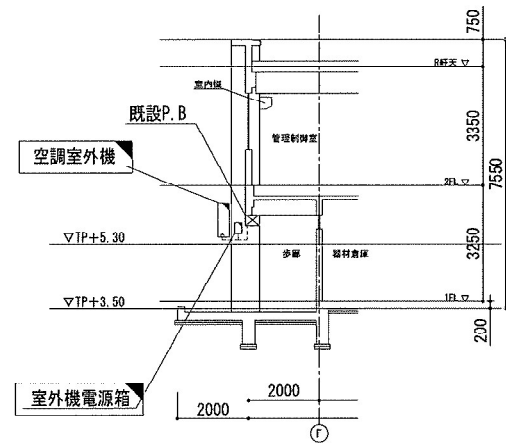
B-B 断面 1/200
