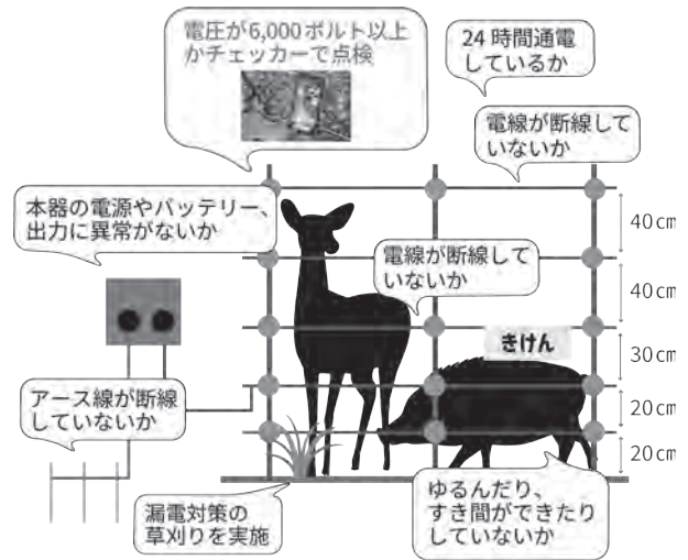
シカ・イノシシ対策の場合 (イノシシのみの場合は、20cm間隔で2段)
